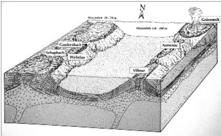
Schematische Darstellung der Region Mittellahn im devonischen Meer
